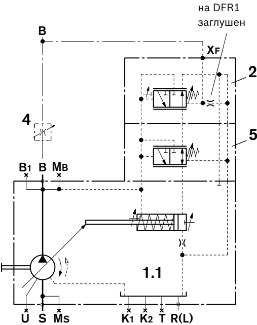
▼ A4VSO, типоразмер 40 и 71
