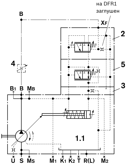
▼ A4VSO, типоразмер 125 – 355
