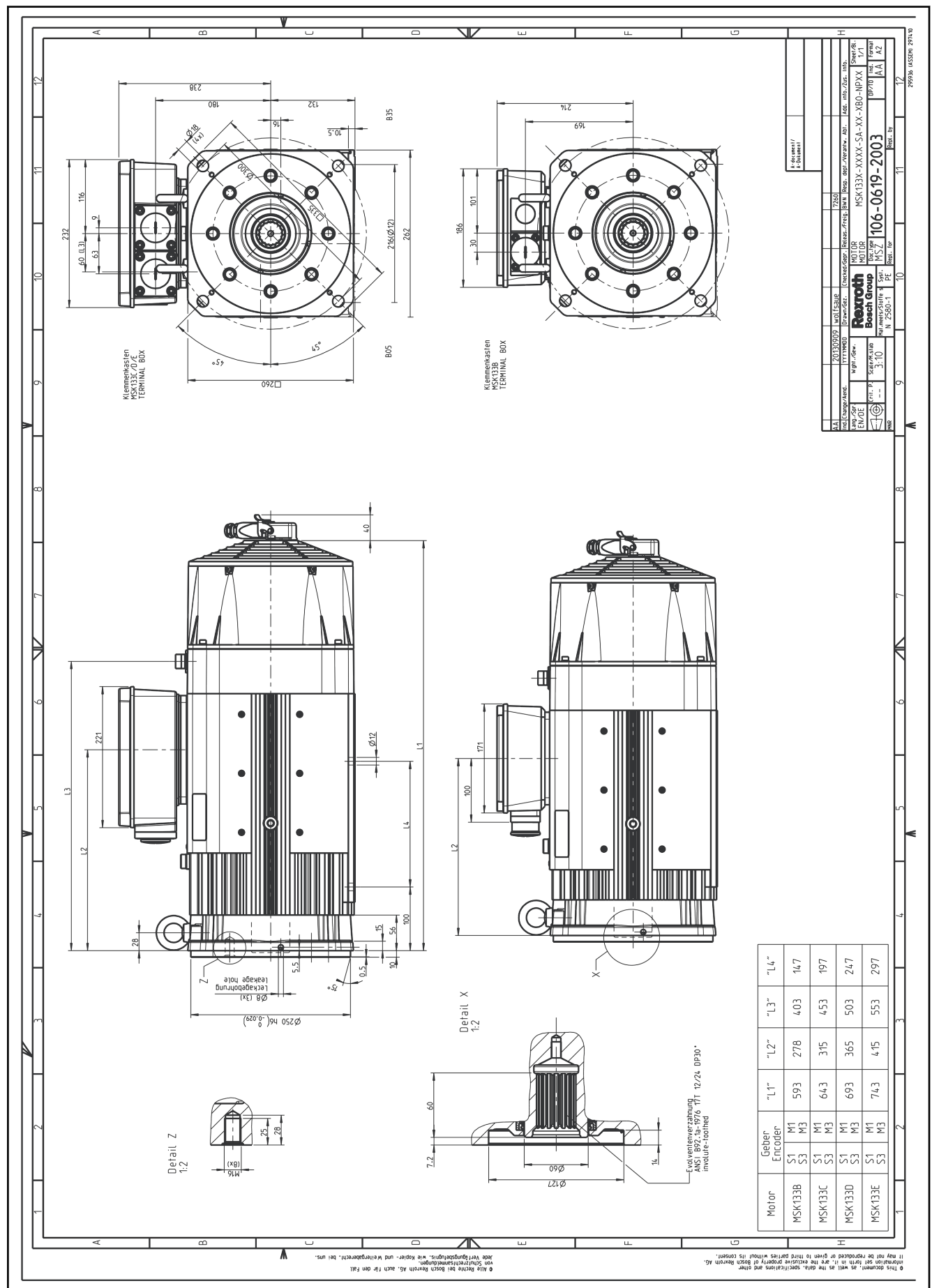
Fig.17-20: MSK133_--SA
